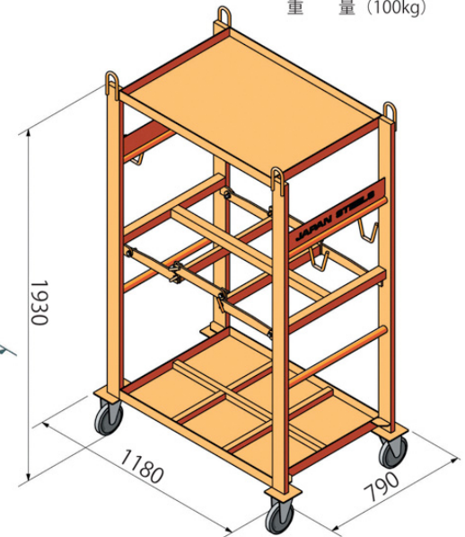
小型ボンベ保管台 G-530B 許容荷重：400kg 重量（100kg）
