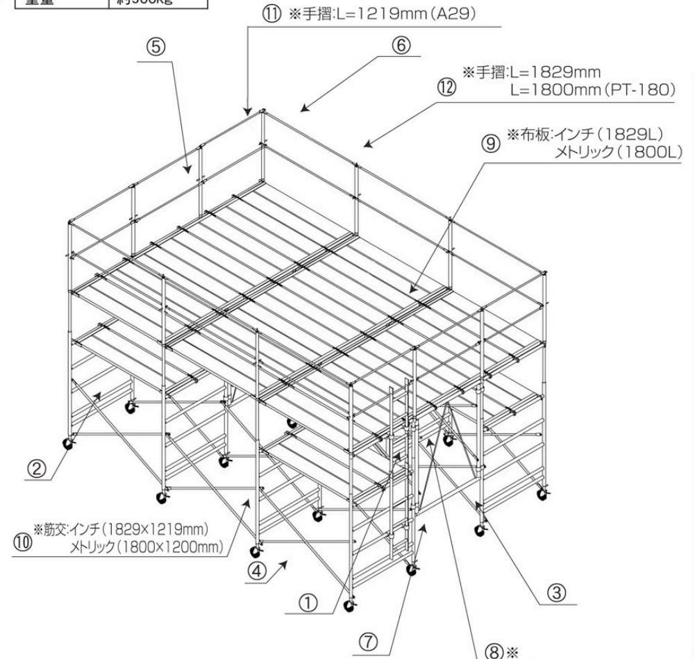
<CP-22/30N 部材表>
