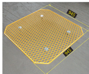
メッシュアクセスカバー 重量(12kg) AC-M945
