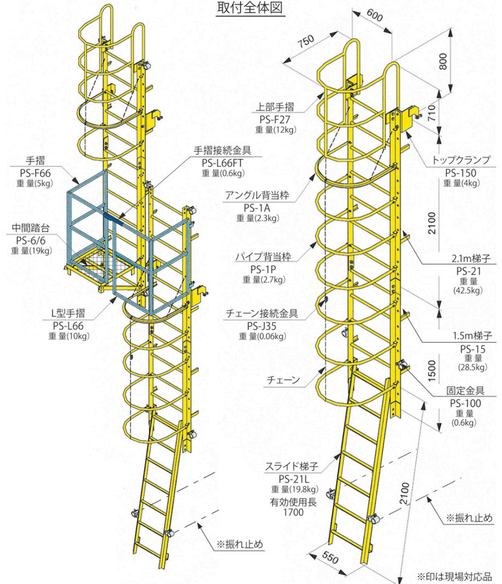
取付全体図
