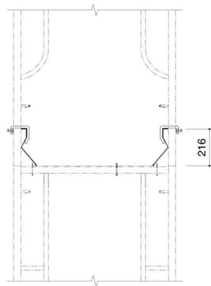
a - a' 矢視図
