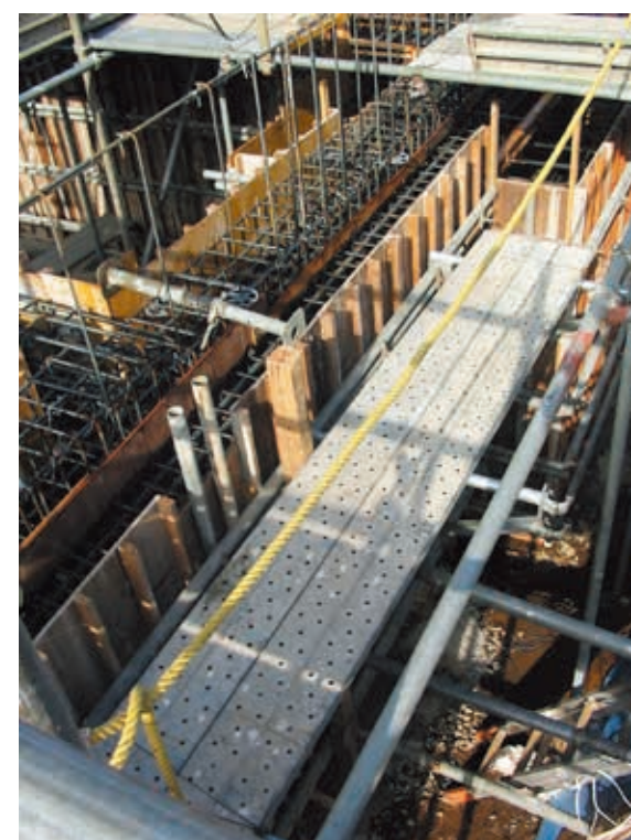
FC-650 足場板(2枚敷)
