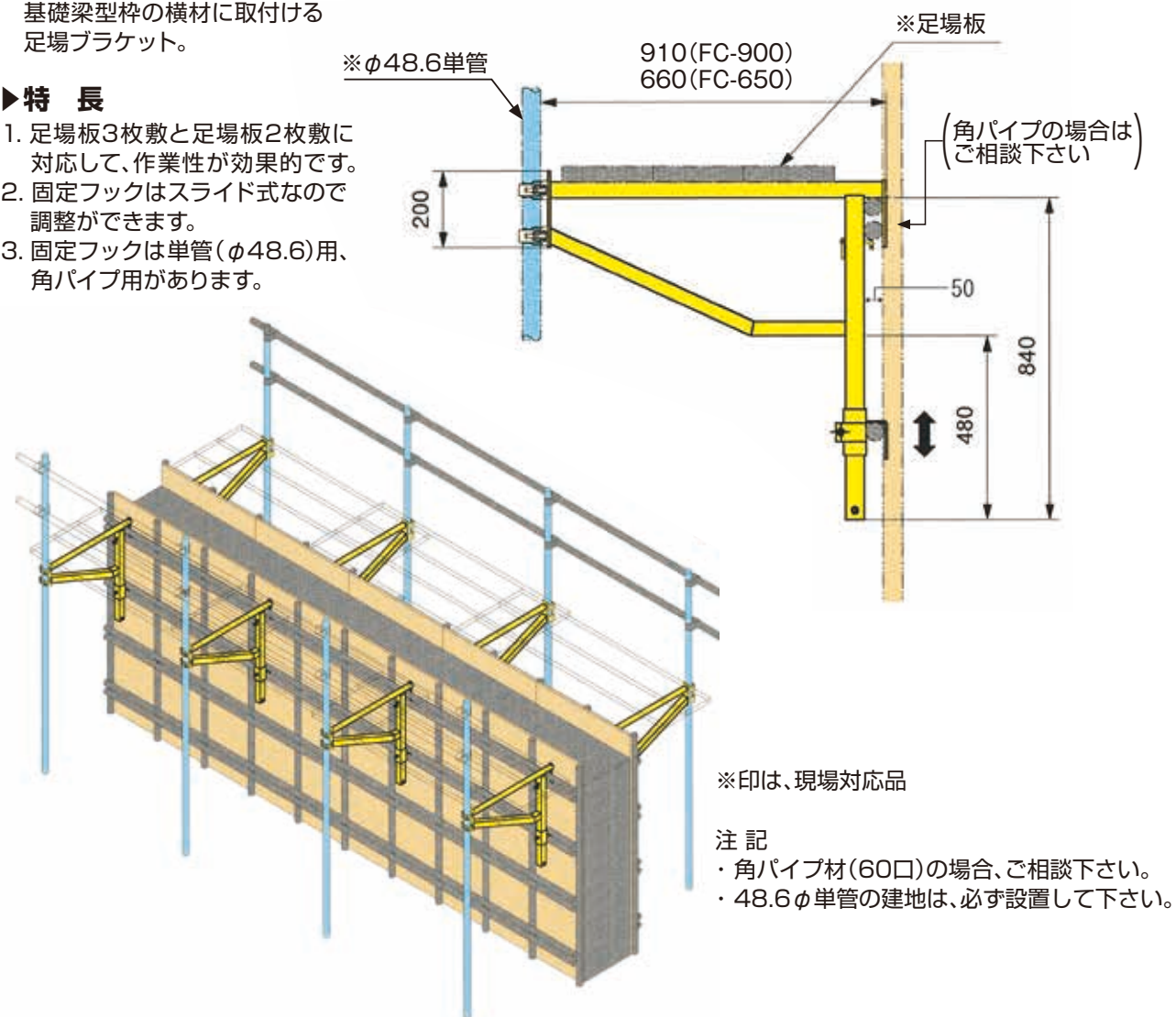
FC-900 足場板(3枚敷)
