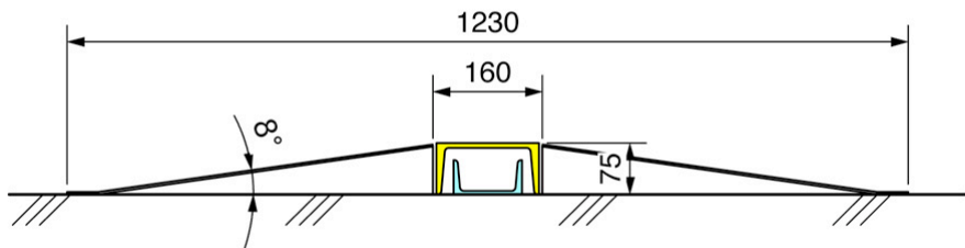
断面図
